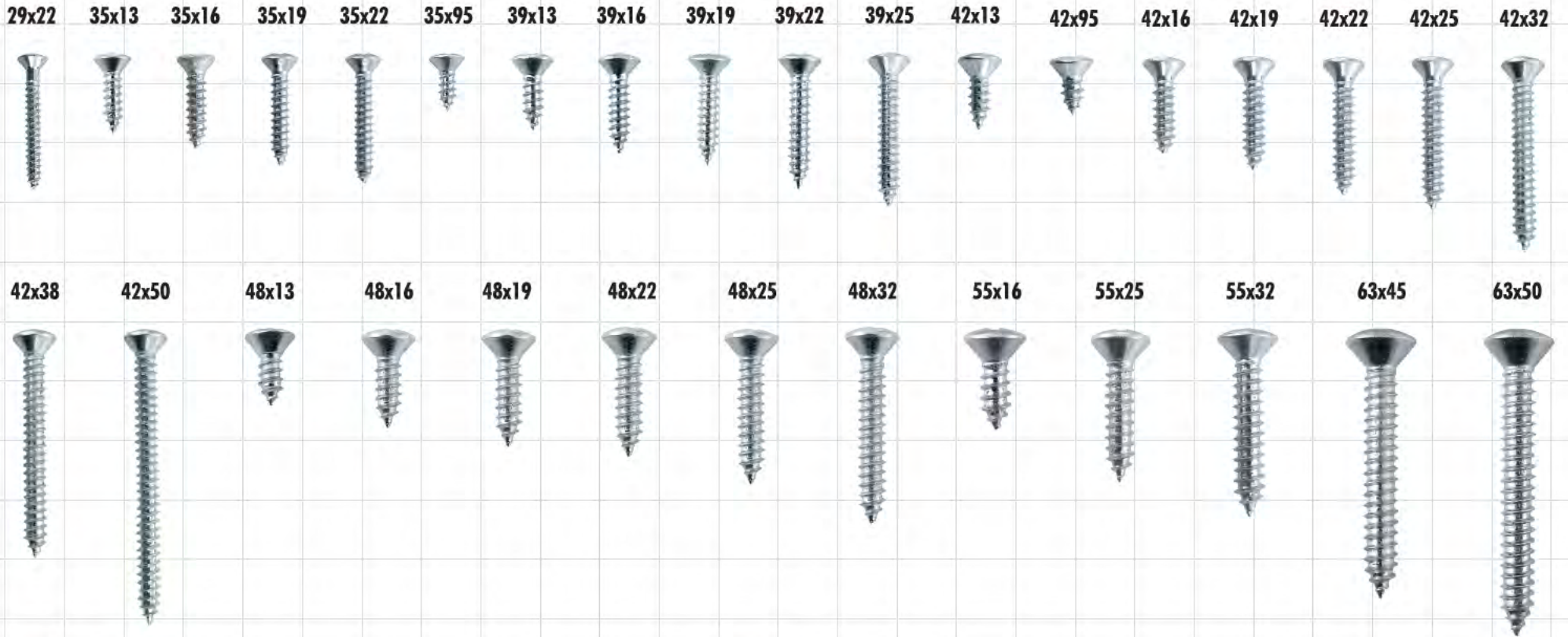
FAMILIA N.º 117 Pija Cónica Cabeza de Gota (Phillips) de Acero Cincado DIN 7983
