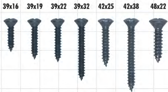
FAMILIA N.º 137 Pija Negra Cónica Cabeza de Gota (Phillips) de Acero Cincado DIN 7983
